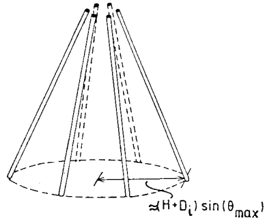
Figur 10.49. Optimal konfiguration då borrhålens maximala lutning är \theta_{\max} och då dessa är borrhåll inom ett litet område vid markytan.
