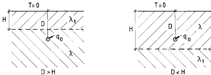
Figur 11.2.8. Stationärt värmeuttag med en slang då marken består av två skikt.
